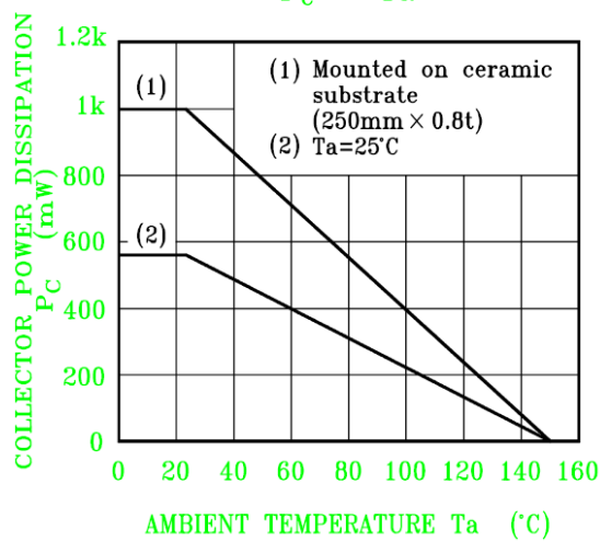
P_C - T_a
